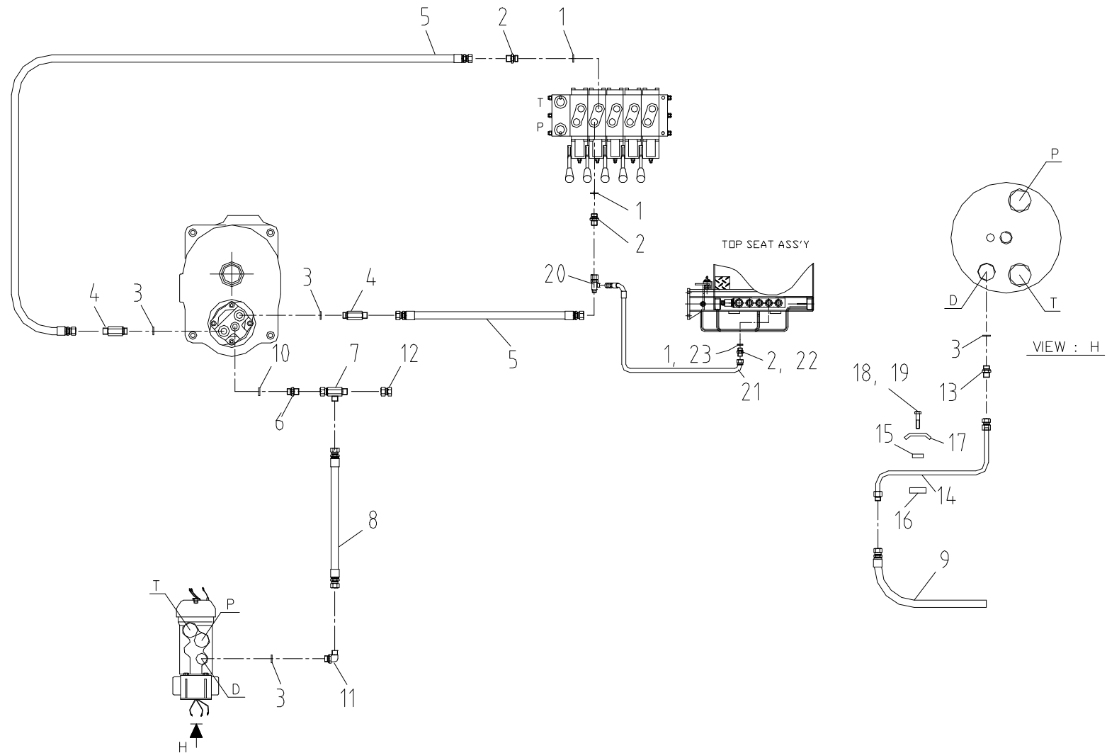
메인 윈치 배관 Fig. 5-3 SCS866LS MAIN WINCH PIPING
