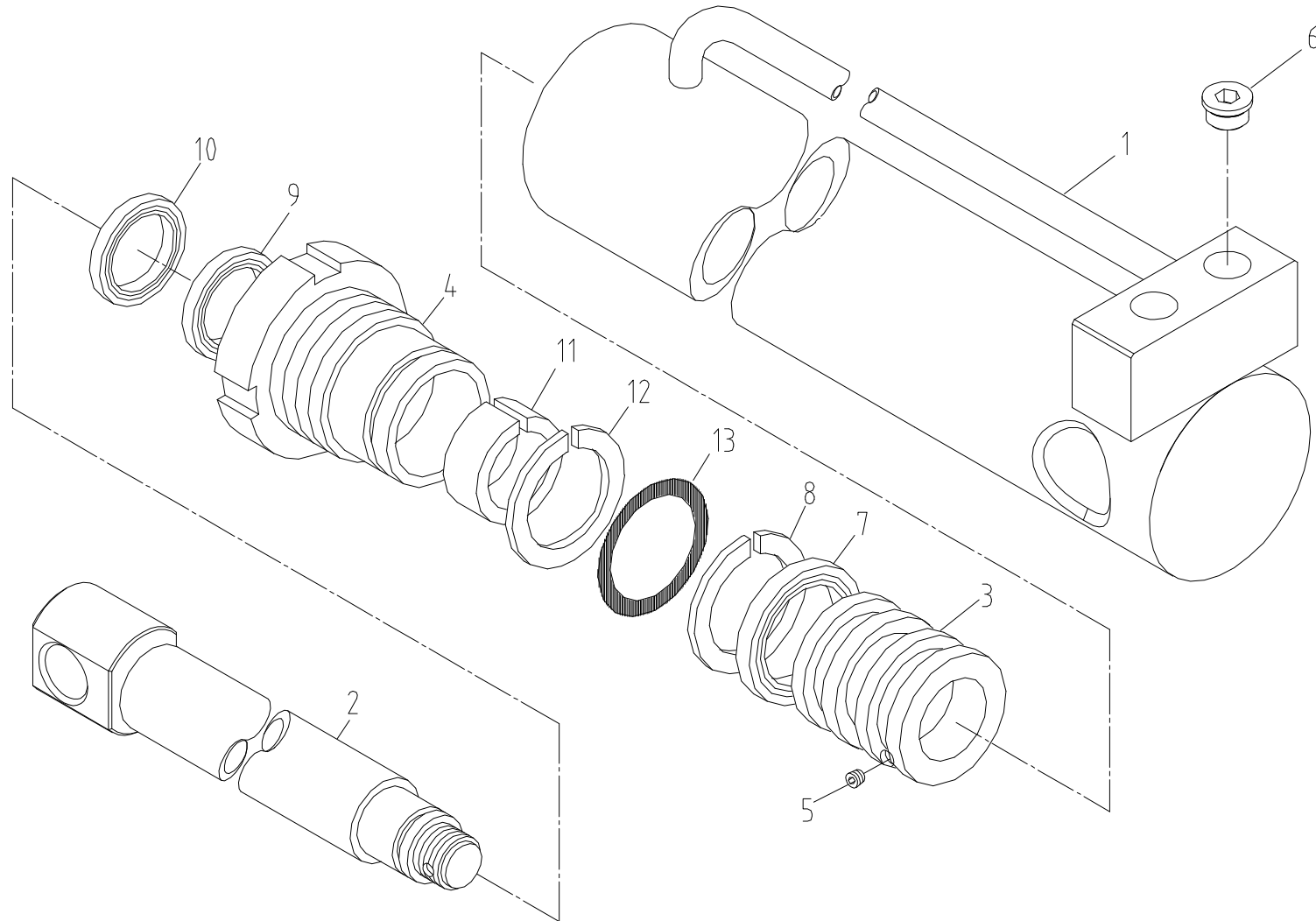
익스펜딩 실린더 조립체 Fig. 4-2 SCS866LS EXPANDING CYL' ASS'Y
