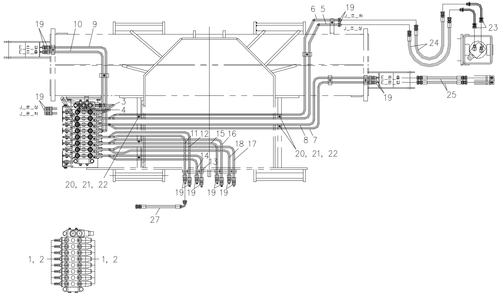
아우트리거 배관 Fig. 5-7 SCS866LS OUTRIGGER PIPING
