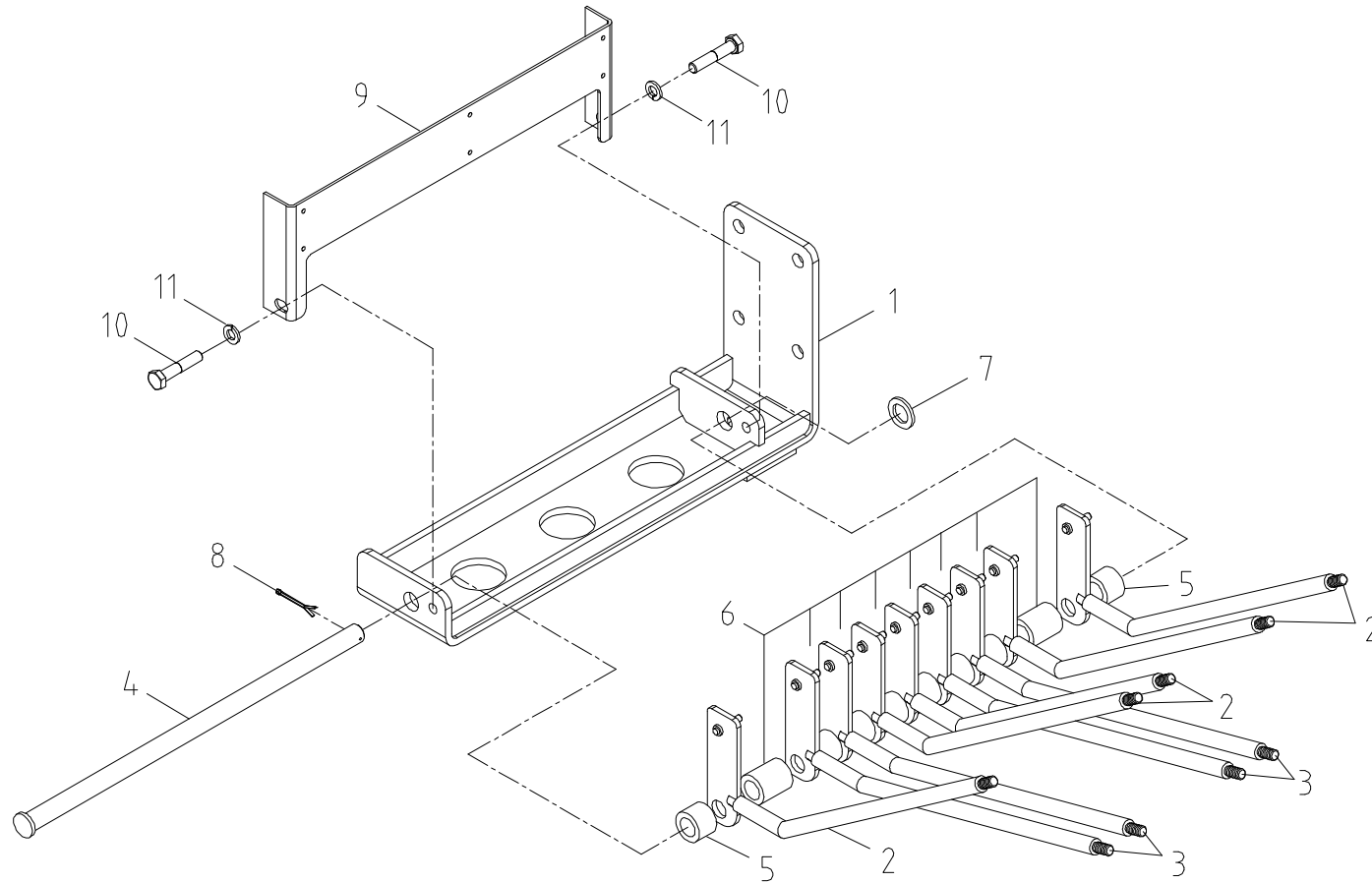
레버 스탠드 셋 Fig. 3-2-2 SCS866LS LEVER STAND SET
