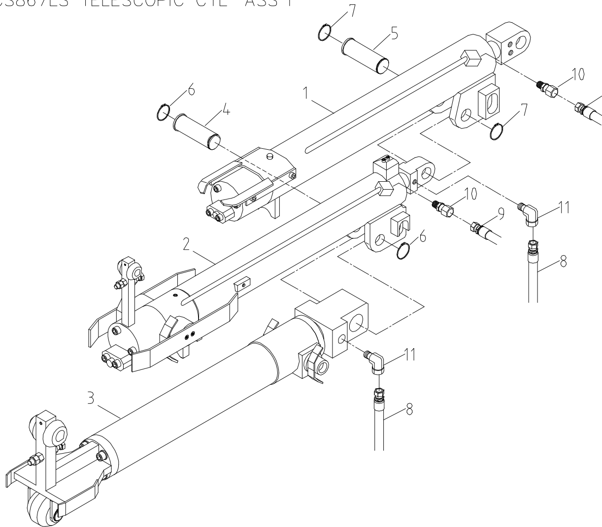
텔레스코픽 실린더 조립체 Fig. 1-1 SCS867LS TELESCOPIC CYL' ASS'Y
