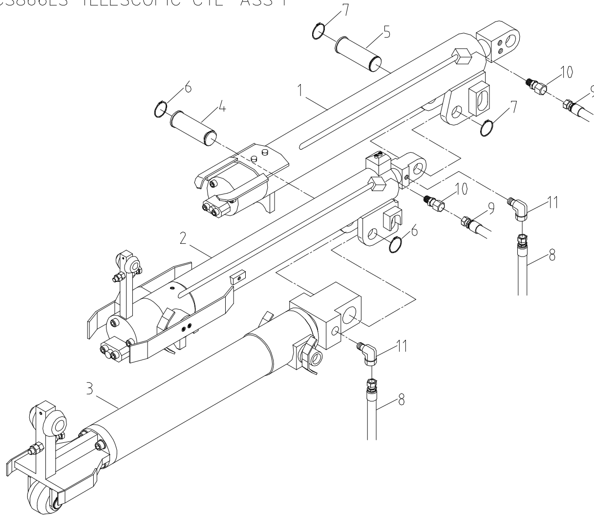
텔레스코픽 실린더 조립체 Fig. 1-1 SCS866LS TELESCOPIC CYL' ASS'Y
