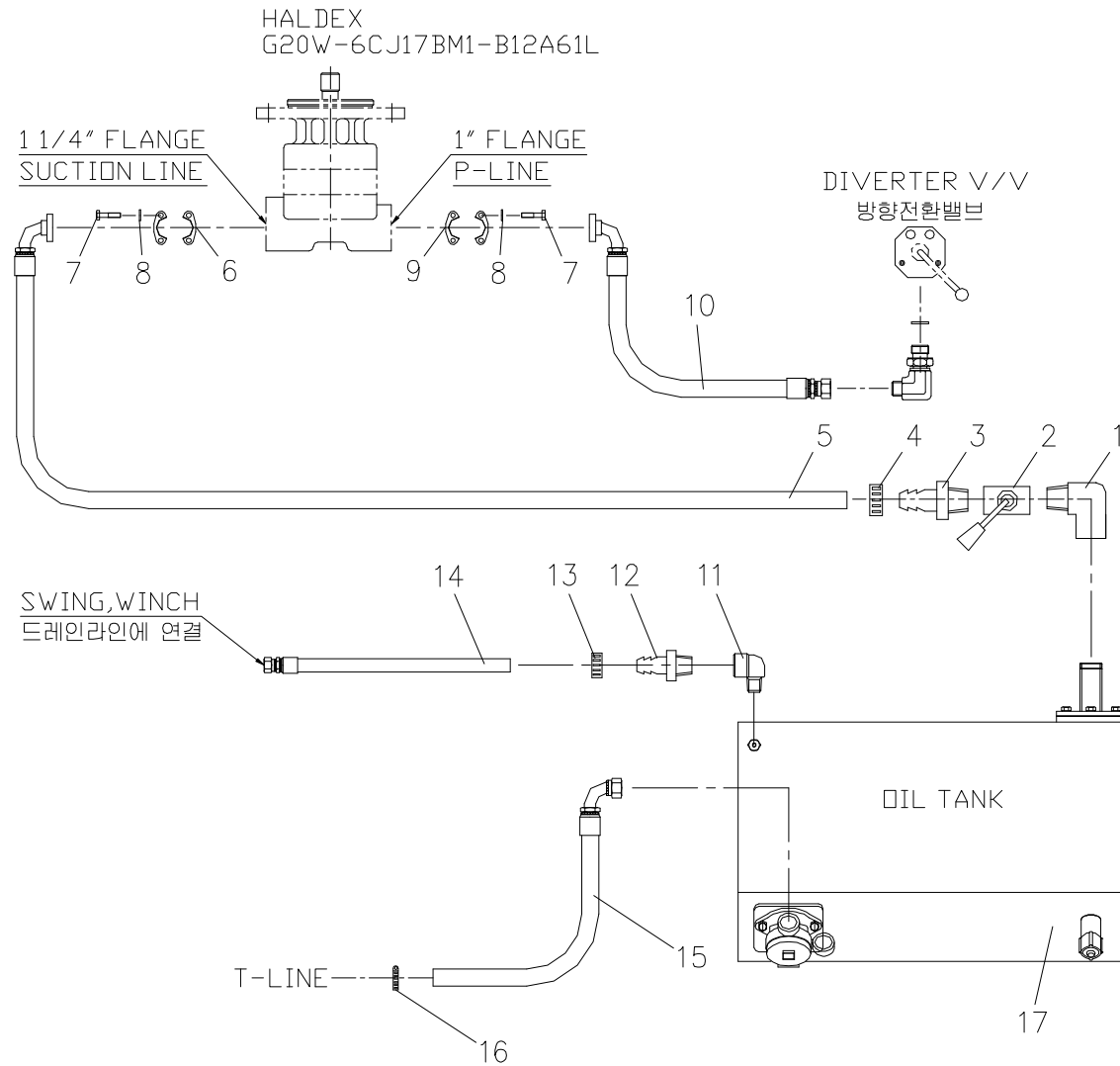
장착 배관 파트 Fig. 9-6 SCS866LS M/T PIPING PART
