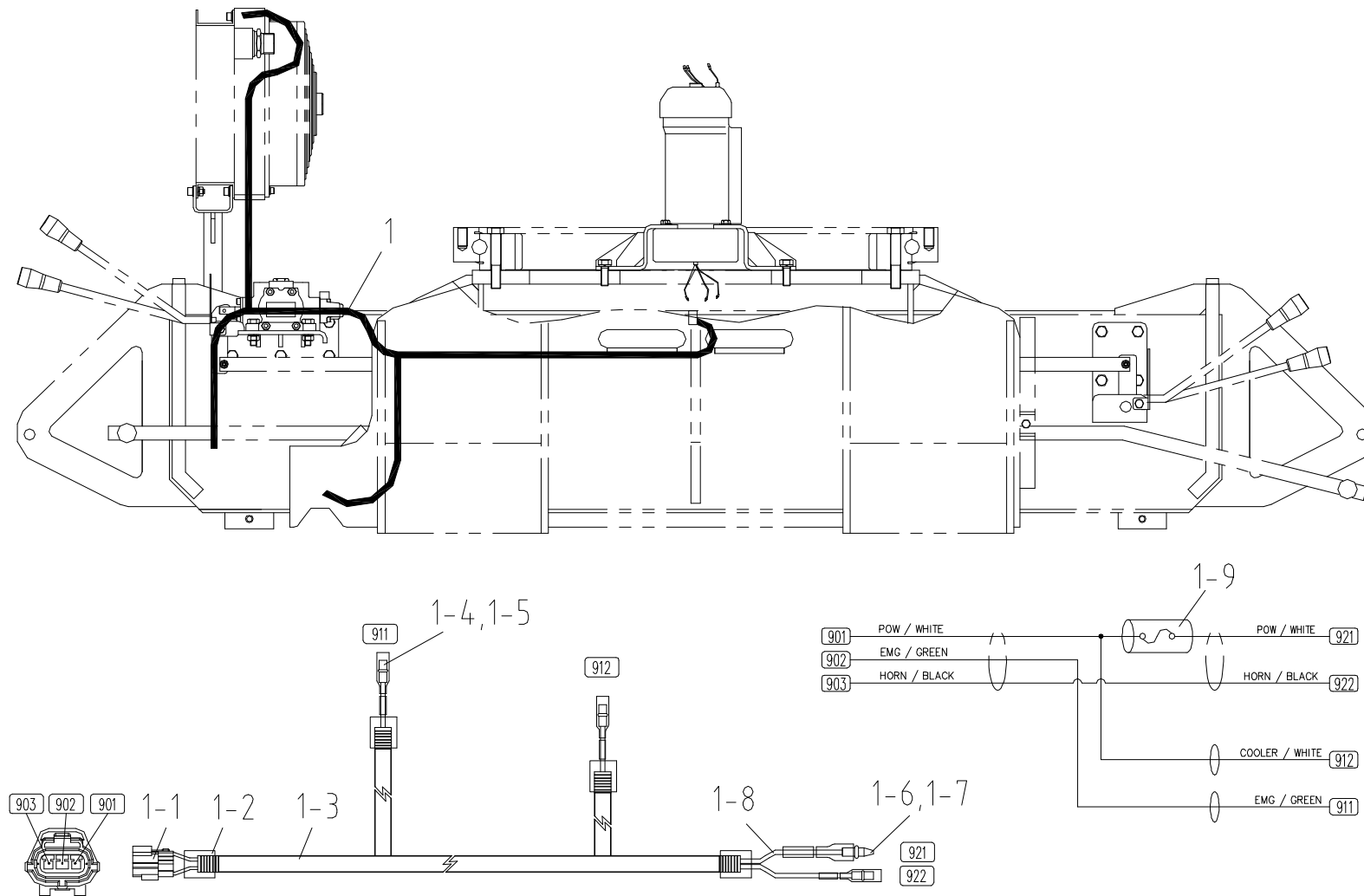
프레임 전선 Fig. 10-1 SCS866LS FRAME WIRING
