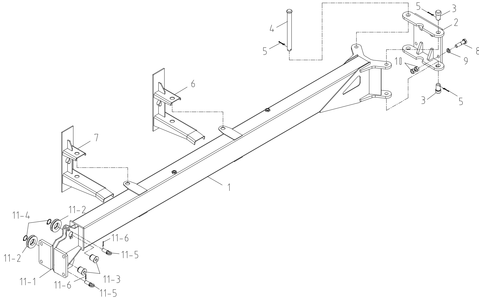
보조 붐 조립체 (3M) Fig. 11 SUB BOOM ASS'Y (3M)
