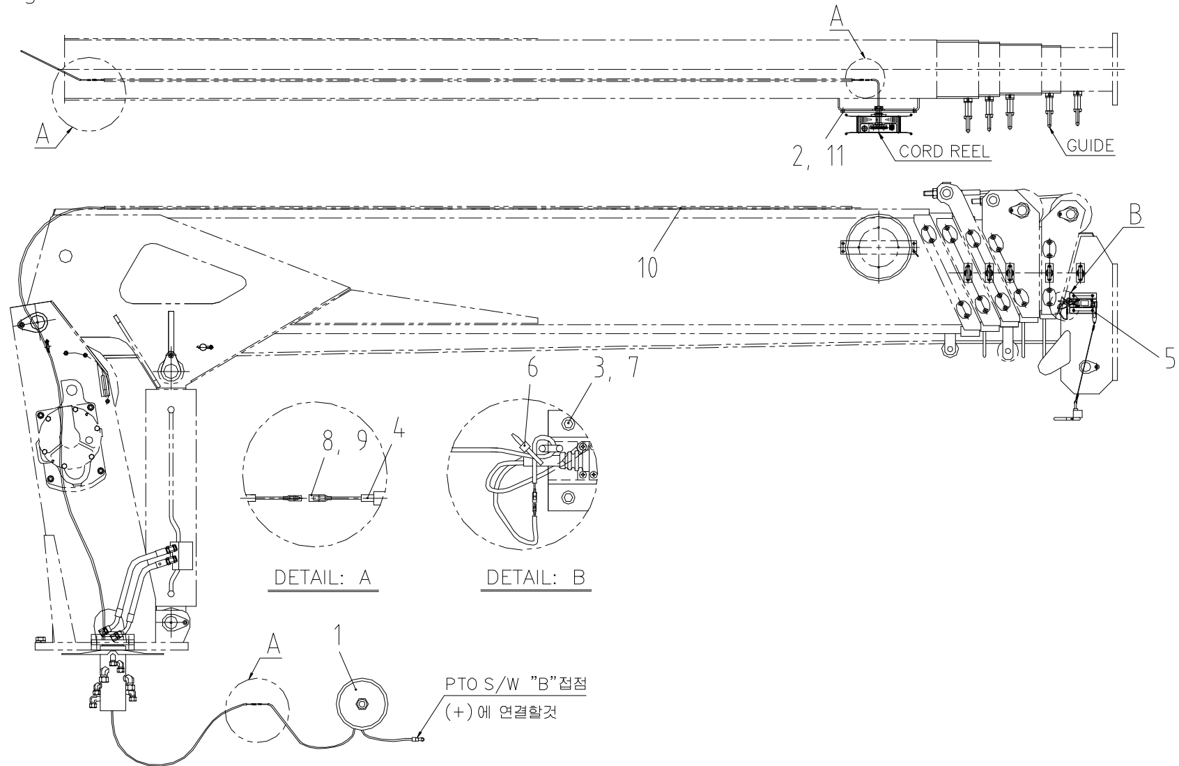
Fig. 14 과권방지장치 조립체
