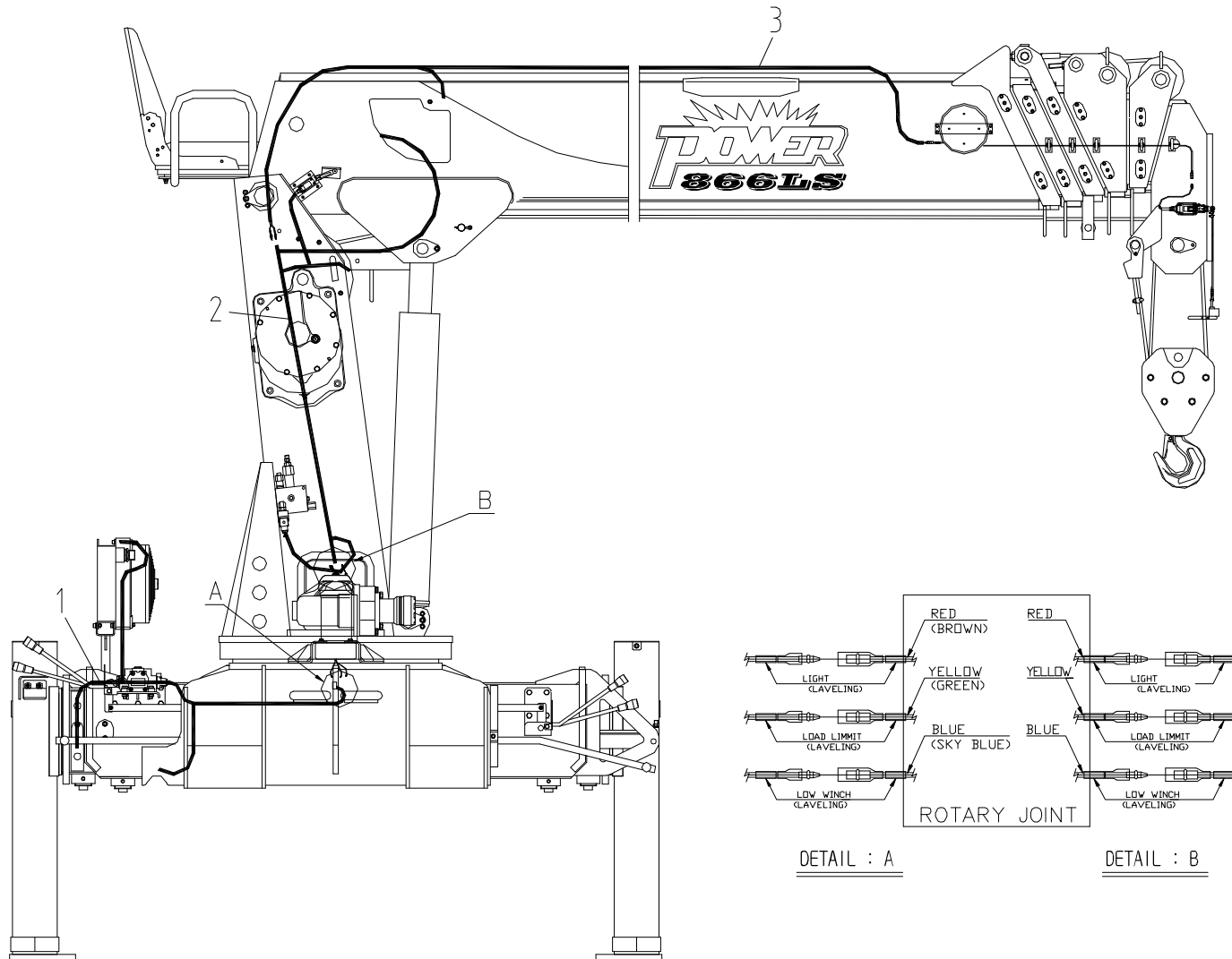
전선 조립체 Fig. 10 SCS866LS WIRING ASS'Y
