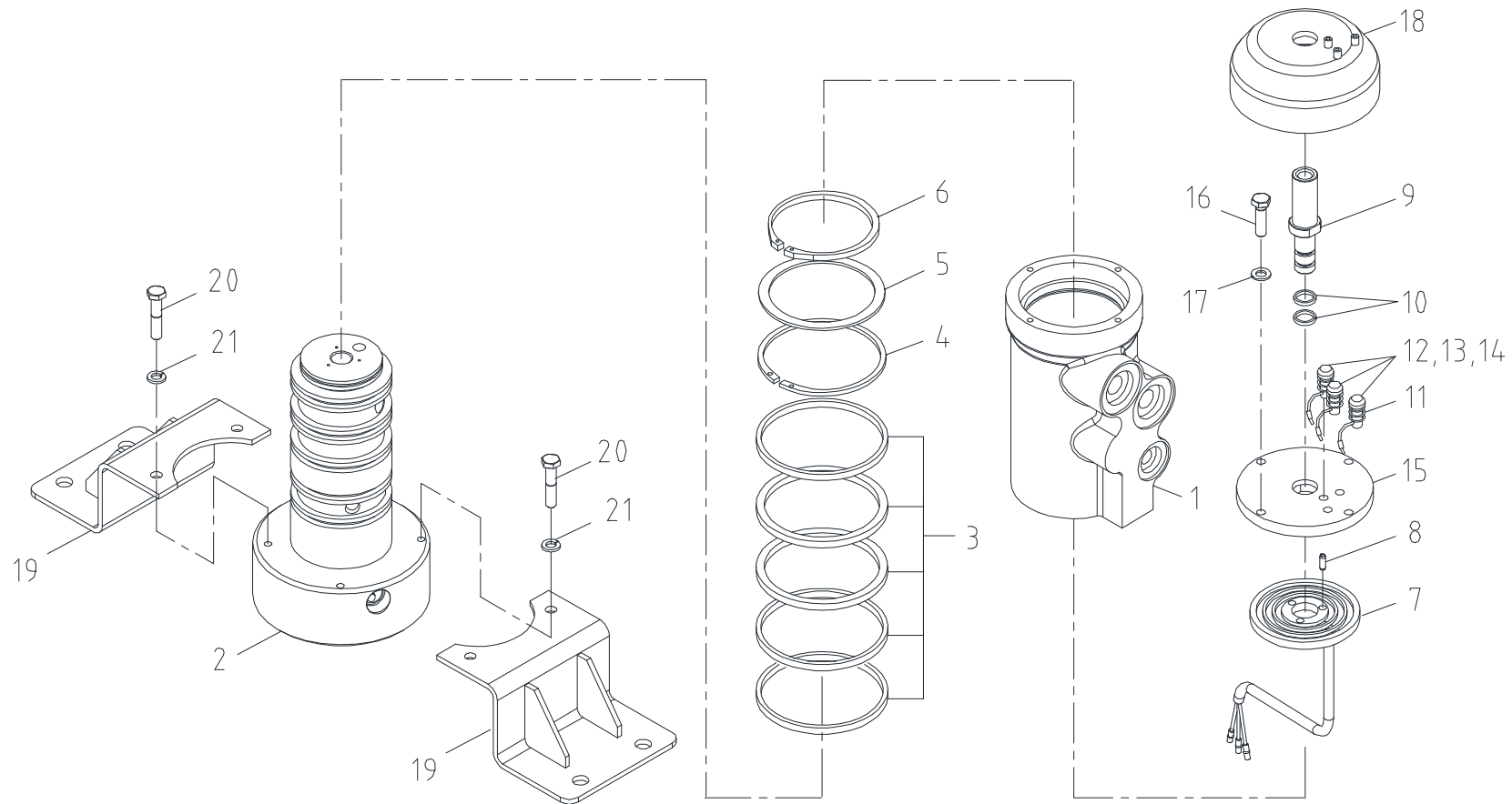
로타리 조인트 조립체 Fig. 3-1 SCS866LS ROTARY JOINT ASS'Y
