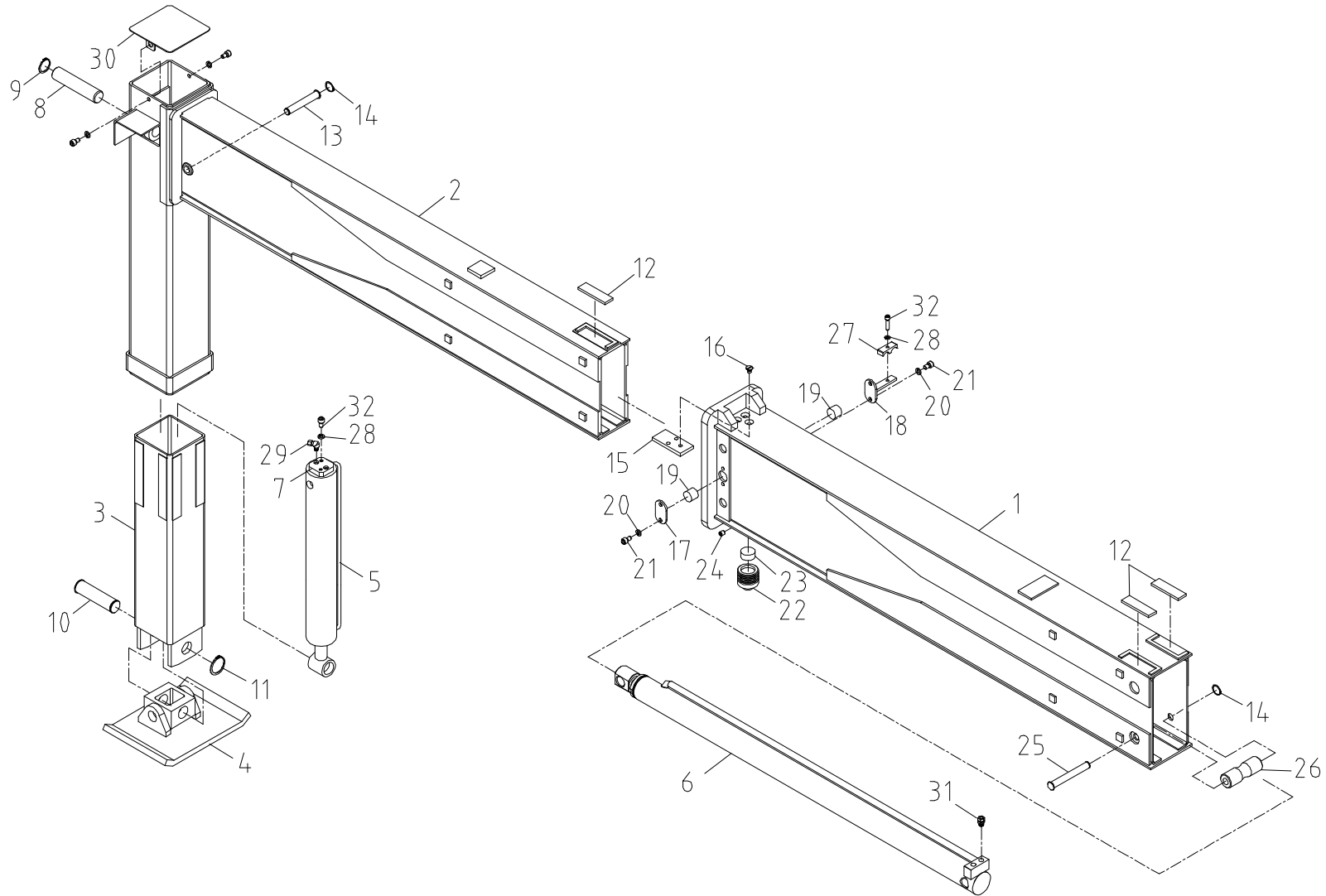
아우트리거 조립체 Fig. 4 SCS866LS OUTRIGGER ASS'Y
