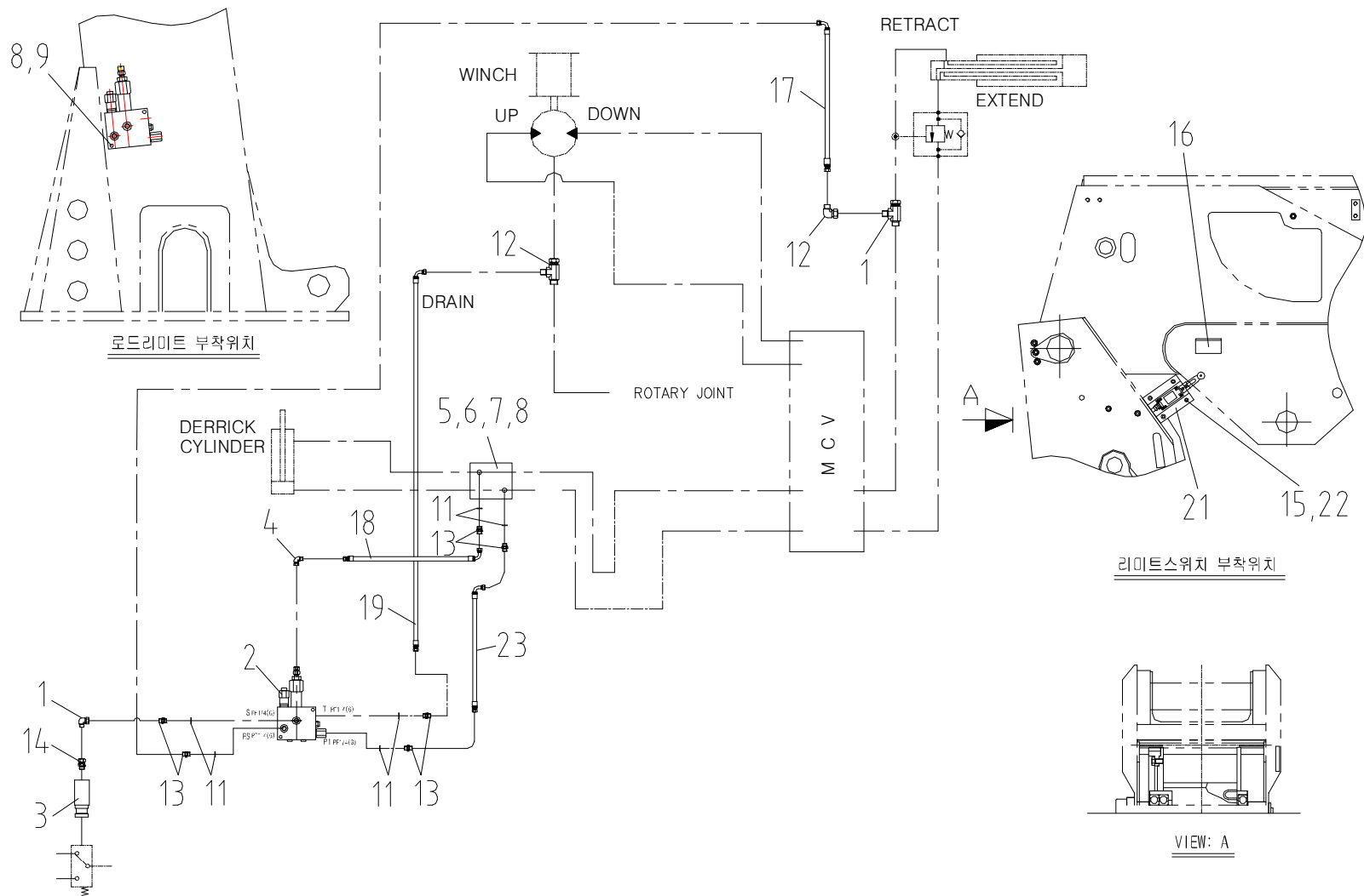
과하중방지 배관 조립체 Fig. 5-8 OVERWINDING ALARM PIPING ASS'Y
