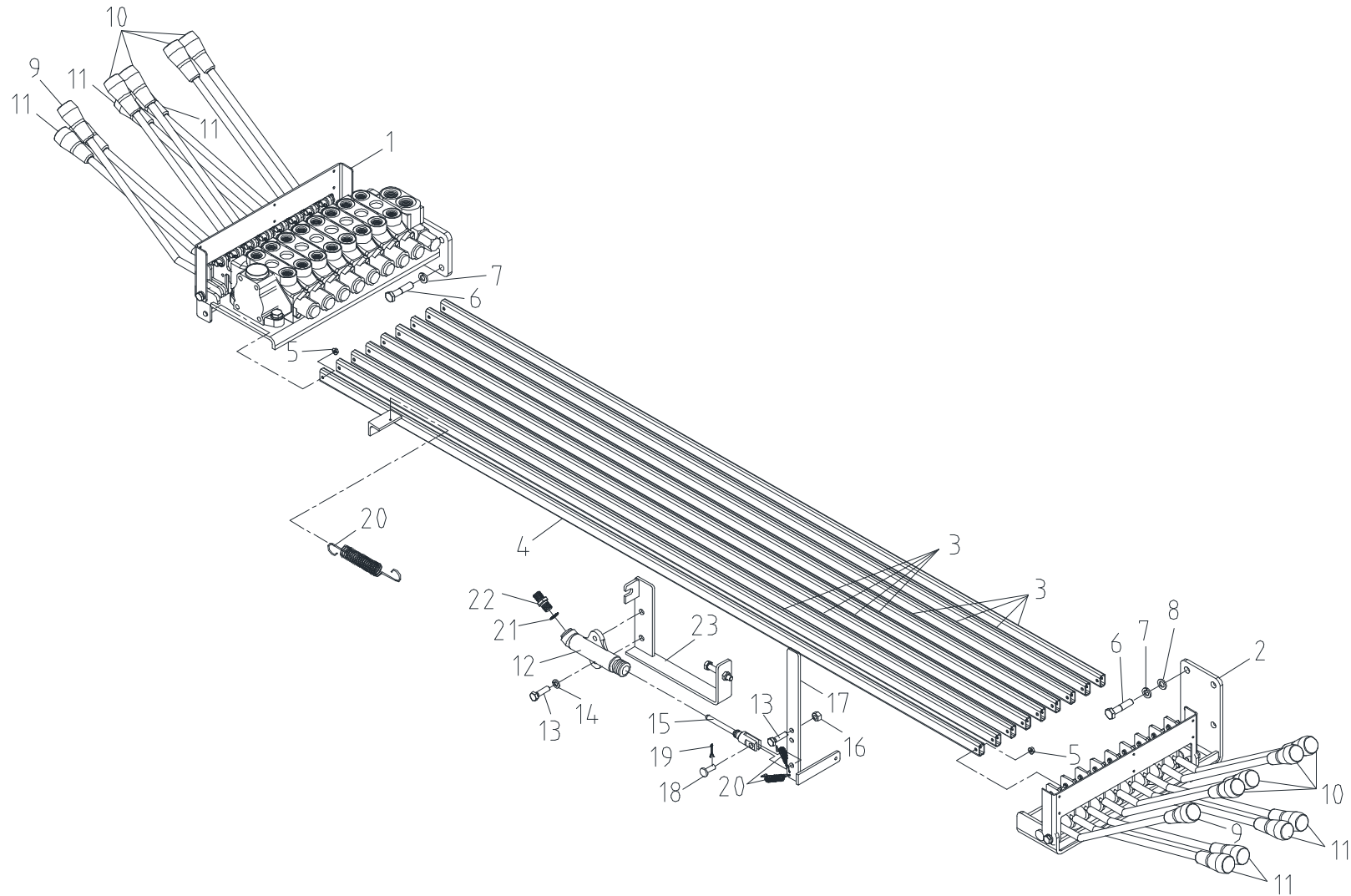
오퍼레이션 조립체 Fig. 3-2 SCS866LS OPERATION ASS'Y
