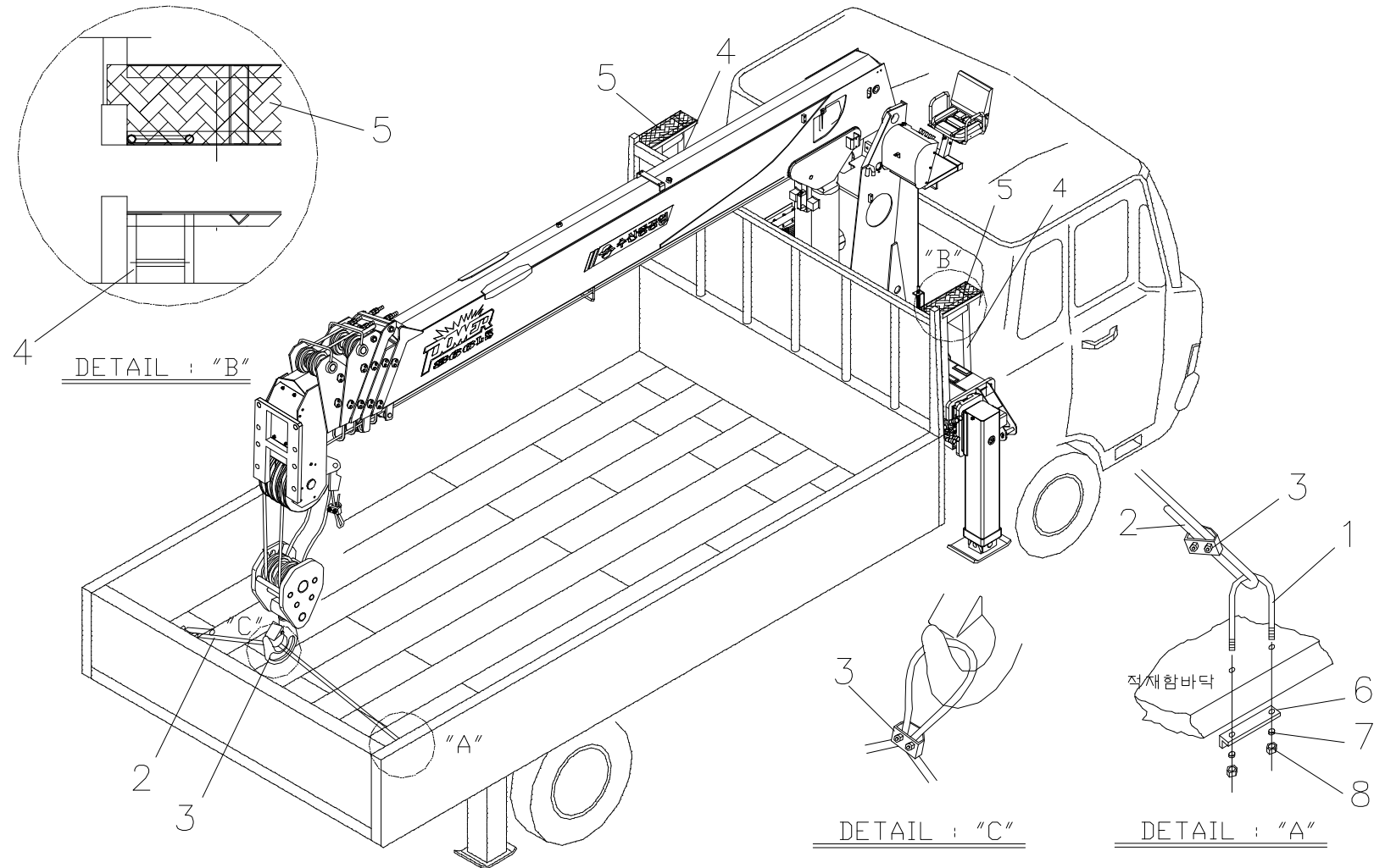
로딩 박스 파트 Fig. 9-5 SCS866LS LOADING BOX PART
