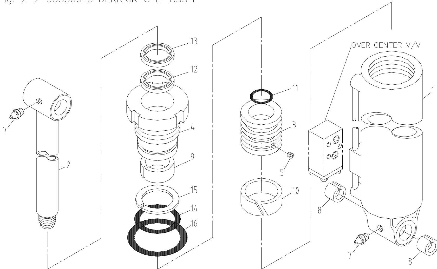
데릭 실린더 조립체 Fig. 2-2 SCS866LS DERRICK CYL' ASS'Y
