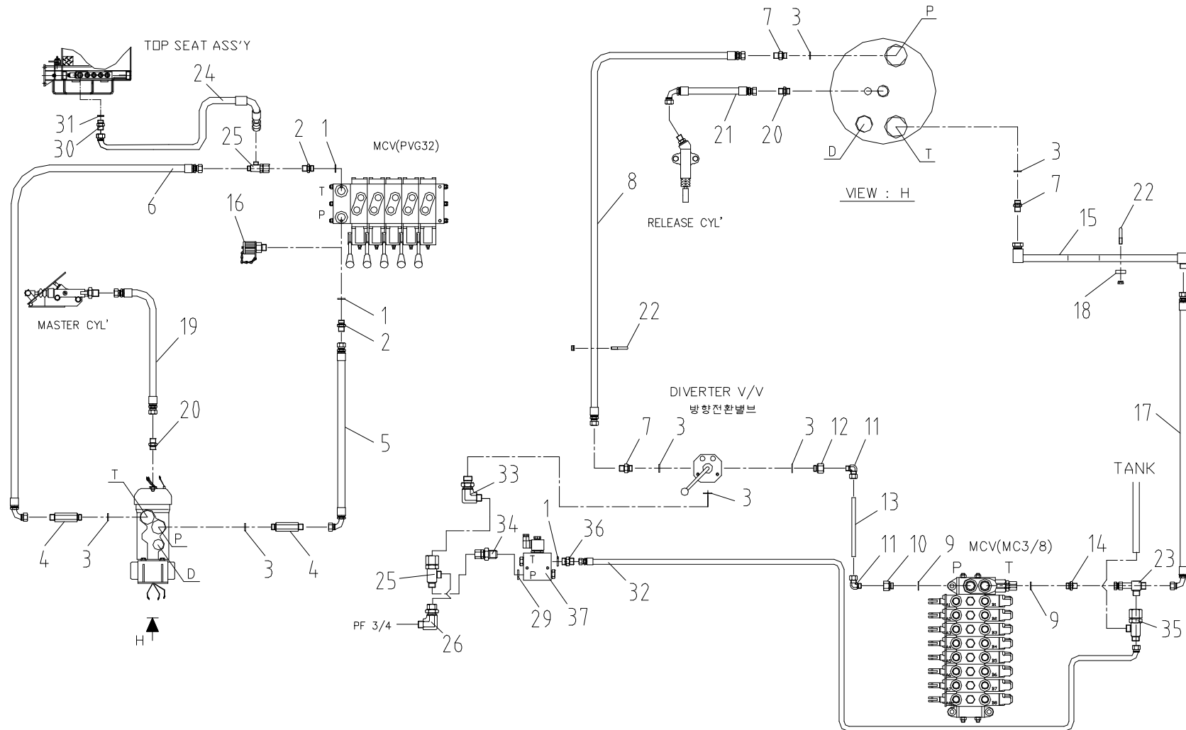
디스트리뷰터 배관 Fig. 5-1 SCS866LS DISTRIBUTOR PIPING
