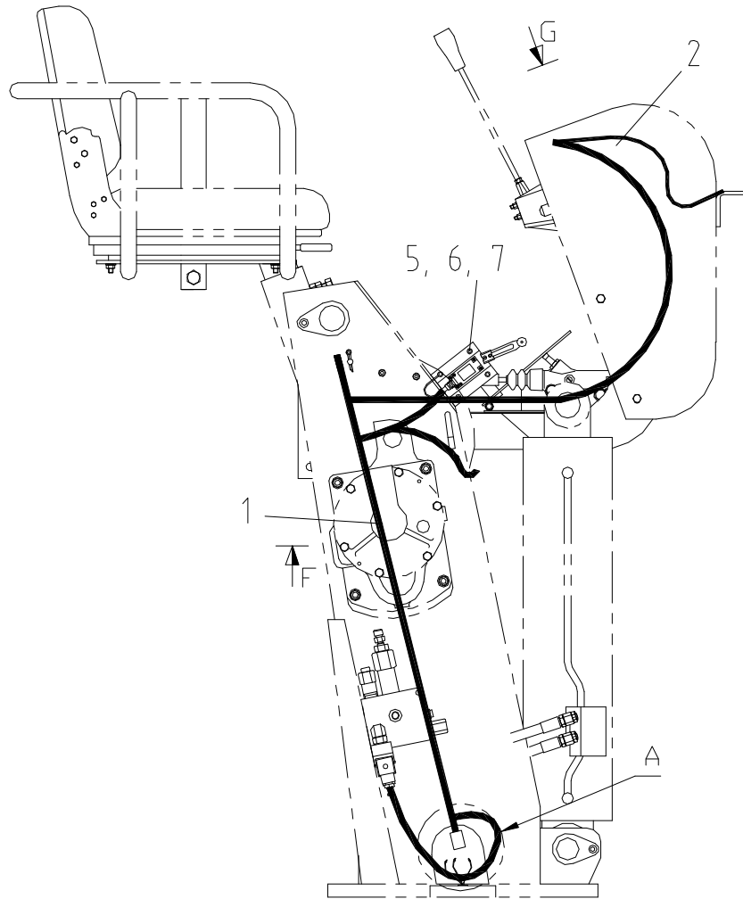
포스트 전선 Fig. 10-2 SCS866LS POST WIRING
