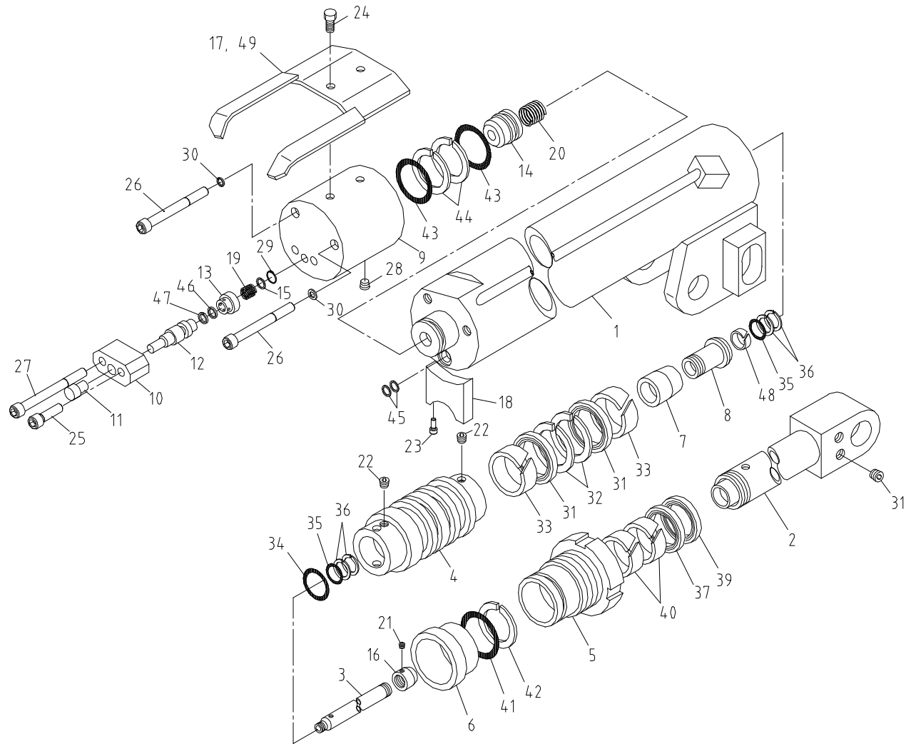
텔레스코픽 실린더(1단) 조립체 Fig. 1-1-1 SCS866LS TELESCOPIC CYL'(1st) ASS'Y
