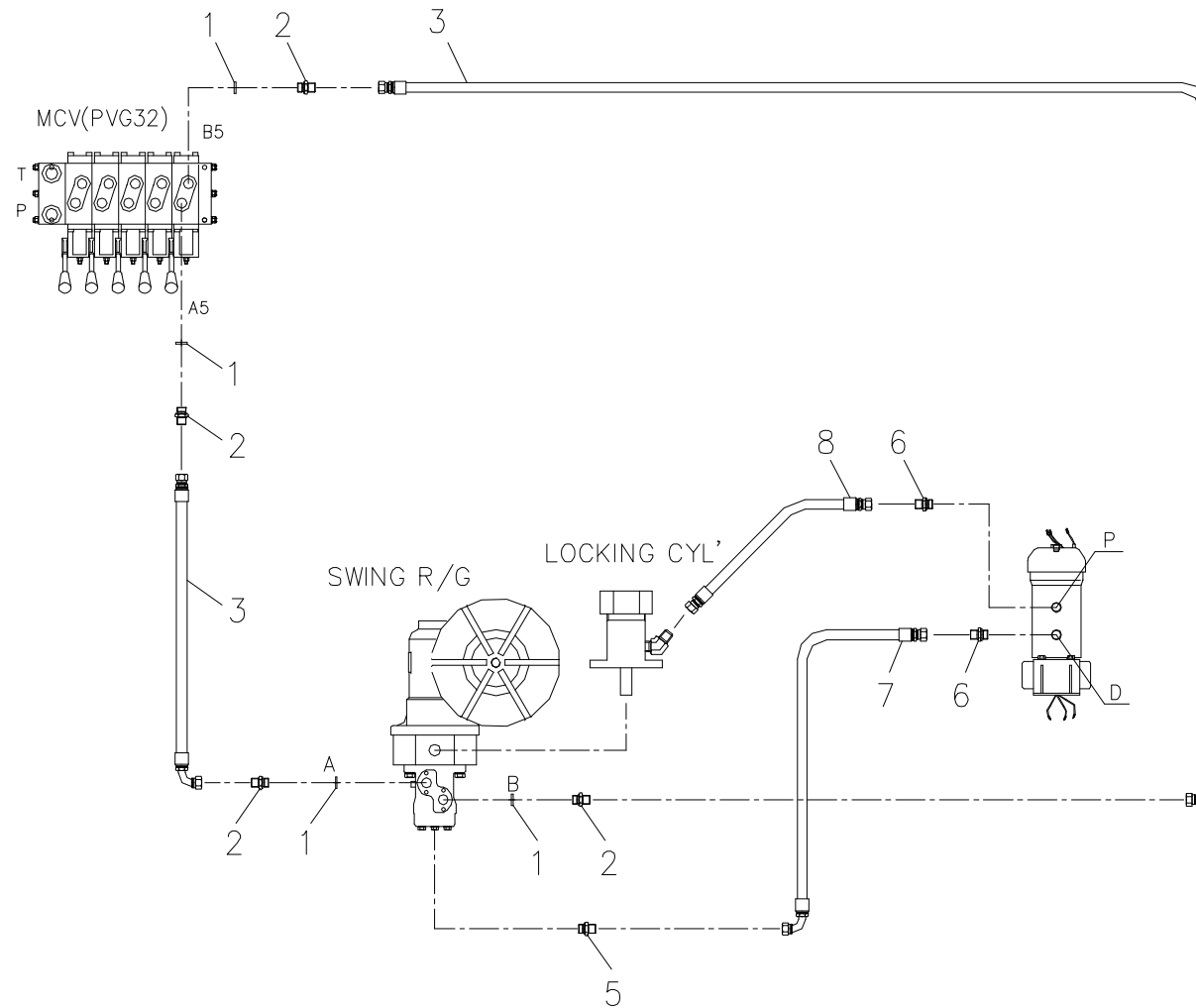
Fig. 5-6 스윙 배관 SCS866LS SWING PIPING
