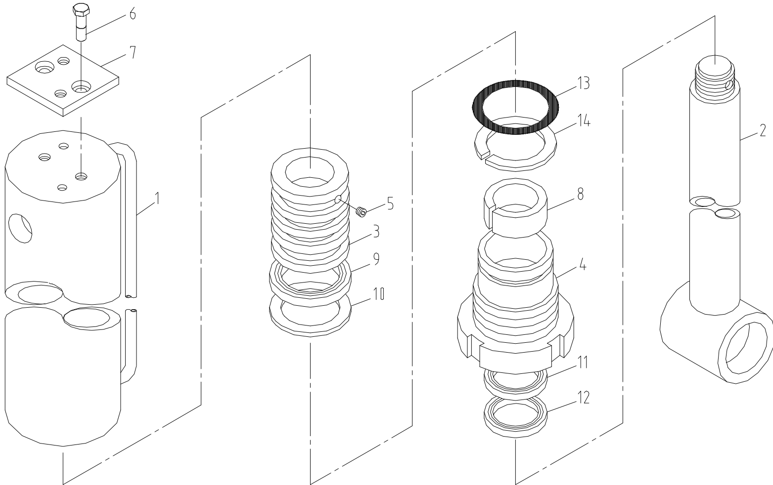
Fig. 4-1 SCS866LS 잭 실린더 조립체 JACK CYL' ASS'Y
