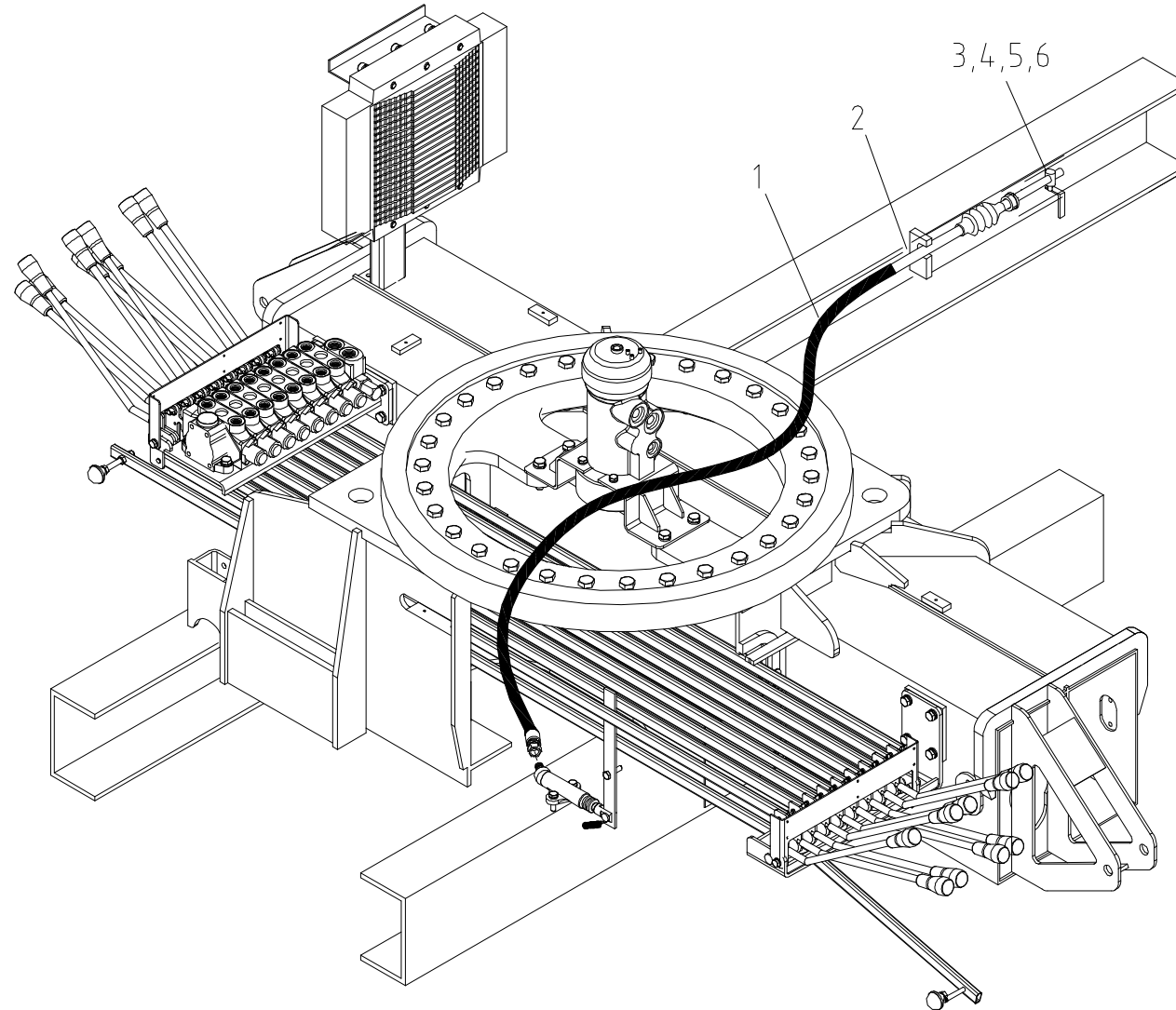
악셀 시스템 파트 Fig. 9-3 SCS866LS ACC'L SYSTEM PART
