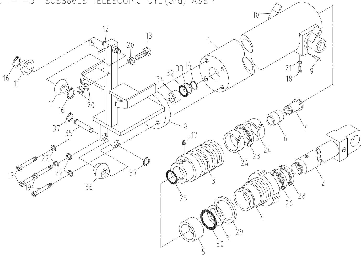
텔레스코픽 실린더(3단) 조립체 Fig. 1-1-3 SCS866LS TELESCOPIC CYL'(3rd) ASS'Y
