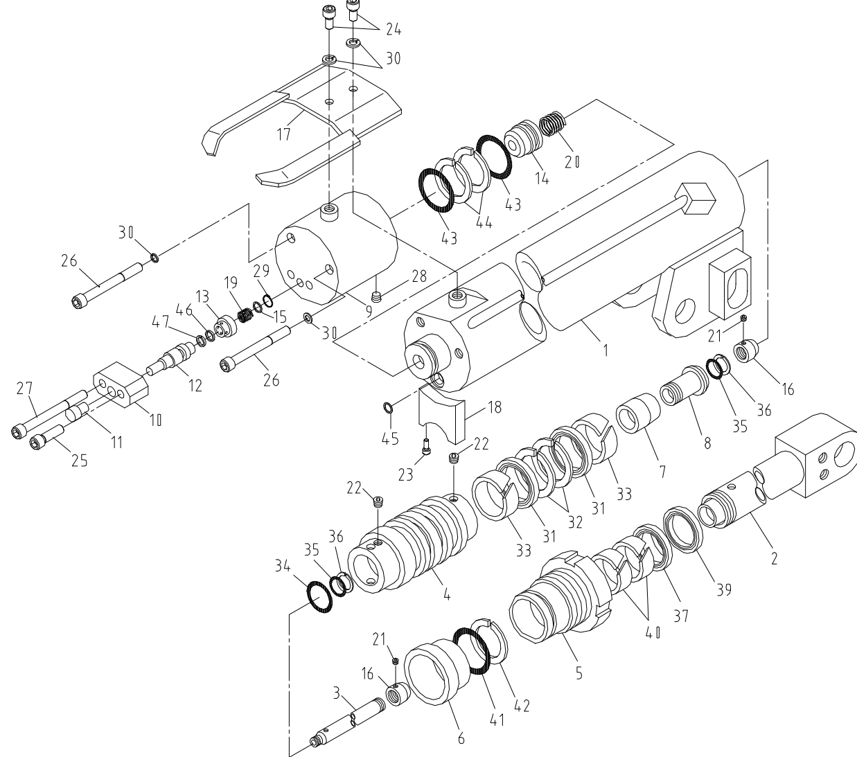
텔레스코픽 실린더(1단) 조립체 Fig. 1-1-1 SCS867LS TELESCOPIC CYL'(1st) ASS'Y
