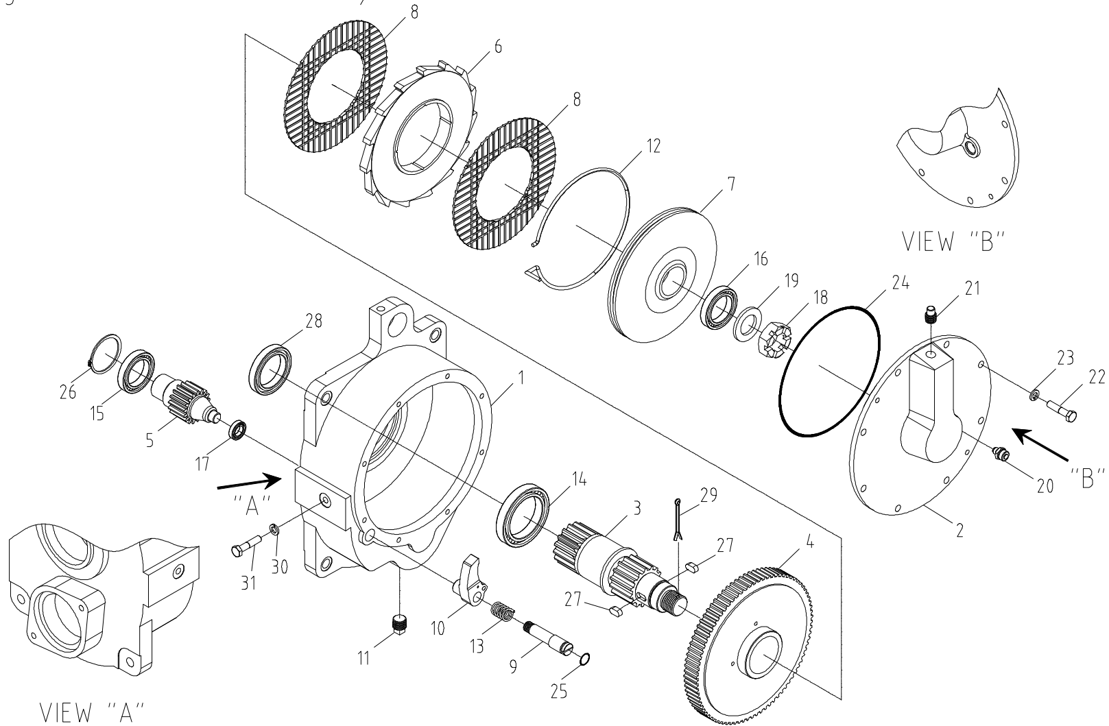
원치 감속기 조립체 Fig. 2-1 SCS866LS WINCH R/G ASS'Y
